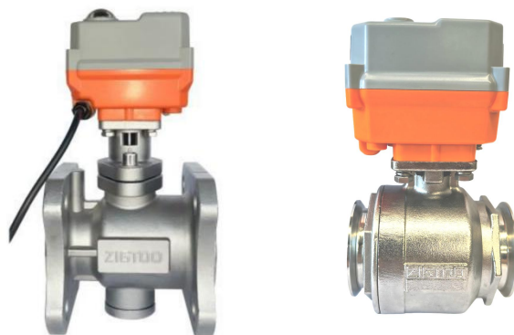
电动调节型球阀 A1003-...系列 PN16
