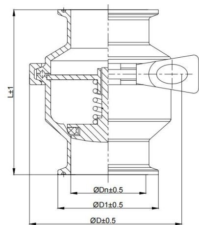
卡盘止回阀
